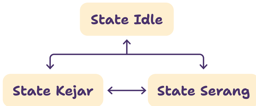
Gambar 4.3 Contoh State yang Merepresentasikan Decision Tree dalam Gim Mr. Alien Sumber: Muhammad Ardhan Fadhlurrahman/Kemendikbudristek (2024)
