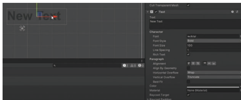
Gambar 4.72 Contoh Implementasi dari UI Text dengan Beberapa Opsi Pilihan Sumber: Muhammad Ardhan Fadhlurrahman/ Kemendikbudristek (2024)
