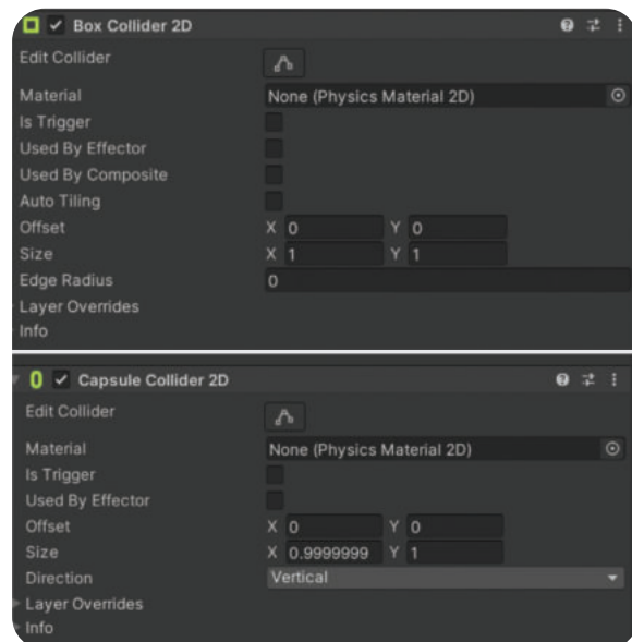
Gambar 5.26 Jenis Implementasi Collider di dalam Game Engine Unity Sumber: Muhammad Ardhan Fadhlurrahman/Kemendikbudristek (2024)
