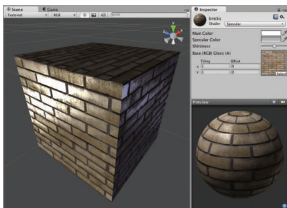
Gambar 5.8 Specular Map di Unity
