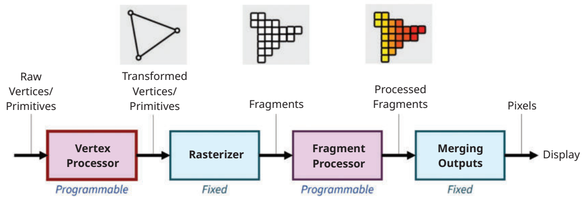
Gambar 5.35 Pipeline Rendering Sebuah Gambar Tiga Dimensi sumber: Youngdo Lee (2024)
