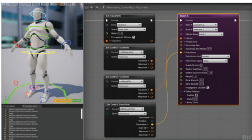
Gambar 5.15 Contoh Automate Rigging dengan Control Rig di Unreal Engine 5 Sumber: Documentation - Control Rig / Epic Games (2024)
