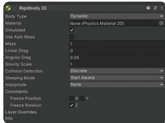
Gambar 5.25 Komponen simulasi fisika bernama Rigidbody 2D Sumber: Muhammad Ardhan Fadhlurrahman/Kemendikbudristek (2024)
