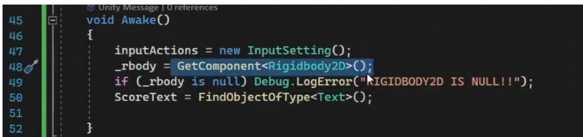
Gambar 4.75 Contoh Implementasi Awake() Tambahan untuk UI Text Sumber: Muhammad Ardhan Fadhlurrahman/ Kemendikbudristek (2024)
