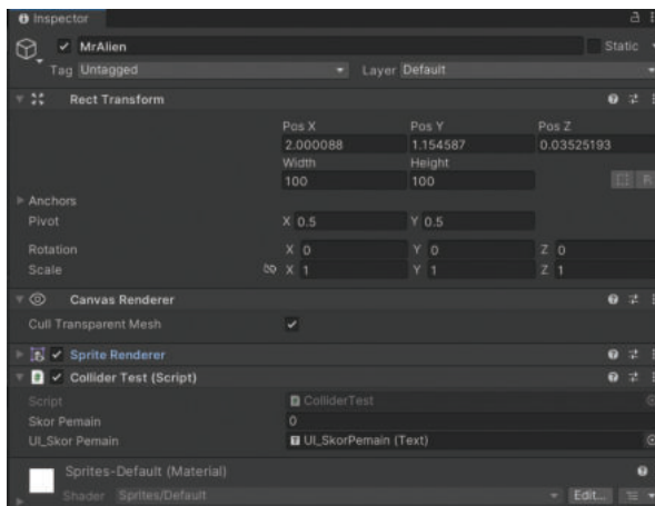
Gambar 4.40 Tampilan Inspector setelah Script dimasukan. Sumber: Muhammad Ardhan Fadhlurrahman / Kemendikbud (2025)
