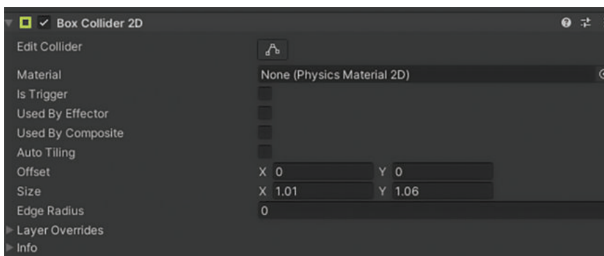
Gambar 4.33 Penjelasan Mengenai Komponen Box Collider 2D Sumber: Muhammad Ardhan Fadhlurrahman/ Kemendikbudristek (2024)
